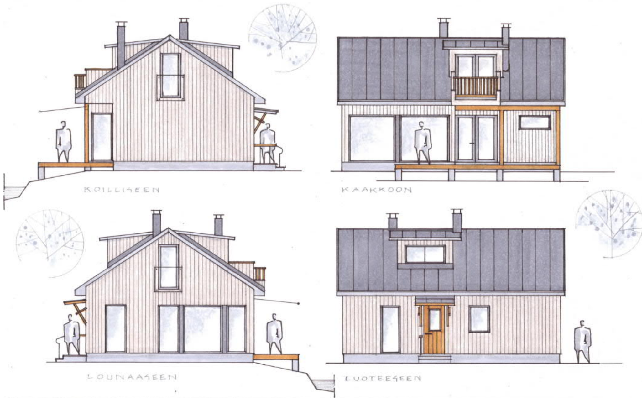
LIITE: Suunnitellun lomarakennuksen julkisivuluonnokset koilliseen, kaakkoon, lounaaseen ja luoteeseen. Arkkitehtuuritoimisto Tiina Vimpari/Tuomo Nakari 30.1.2023
